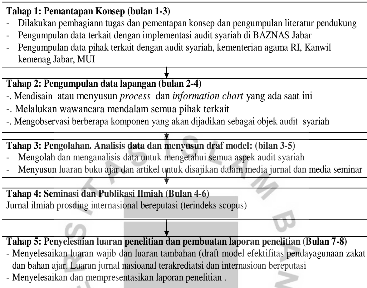
Gambar 4.1 Tahap-Tahap Penelitian
